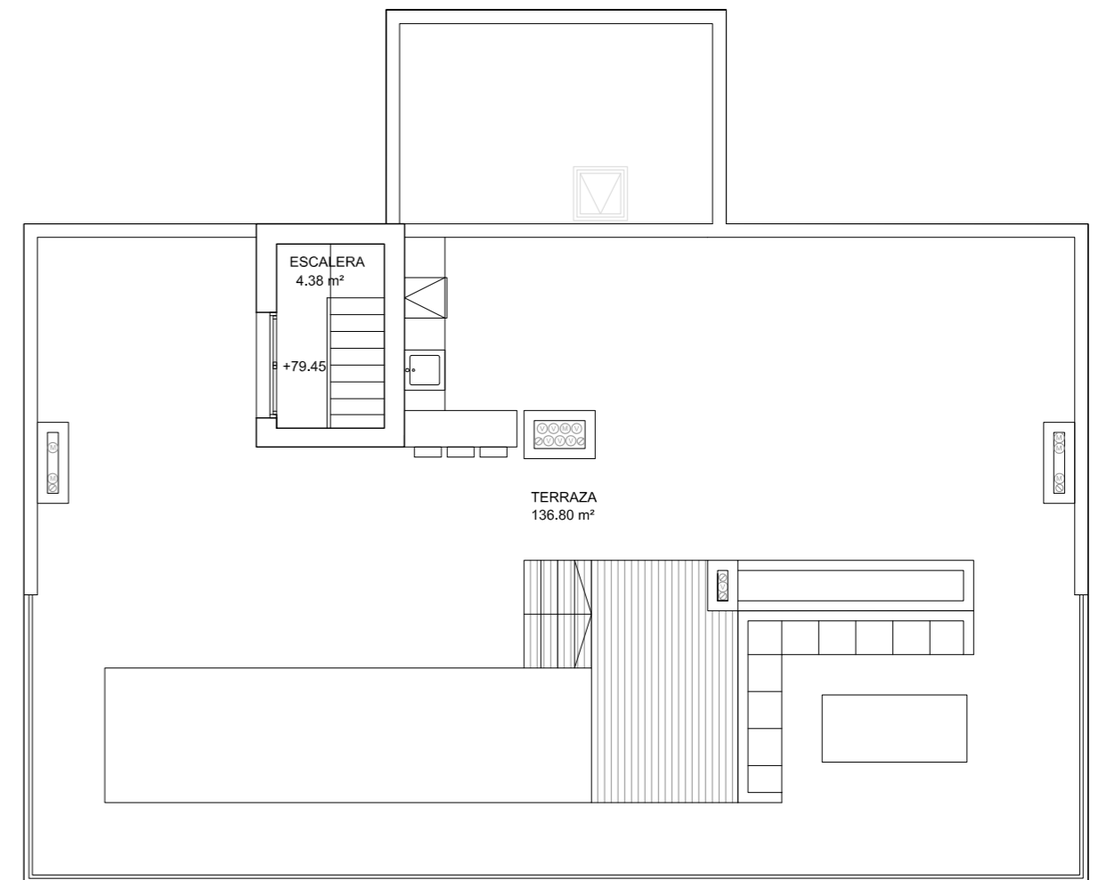
Planta Cubierta
