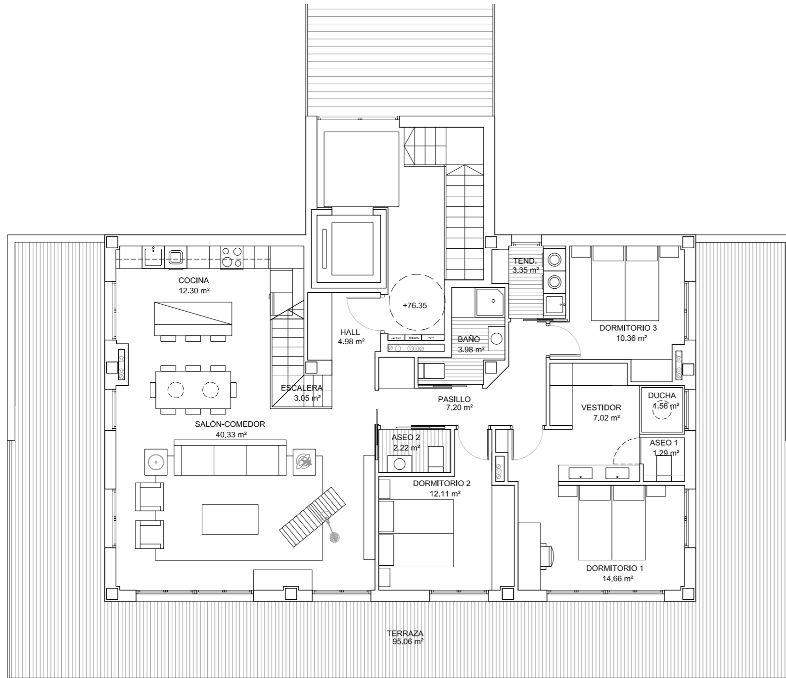
Planta Segunda
