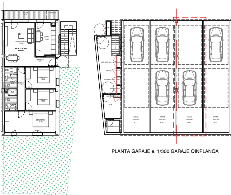
PLANTA VIVIENDA e. 1/100, 1/300 ETXEBIZITZAREN OINPLANOA
