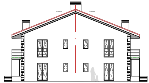
ALZADO ALKAIGA ERDIA e. 1/300 ALKAIGA ERDIA ALTXAERA
